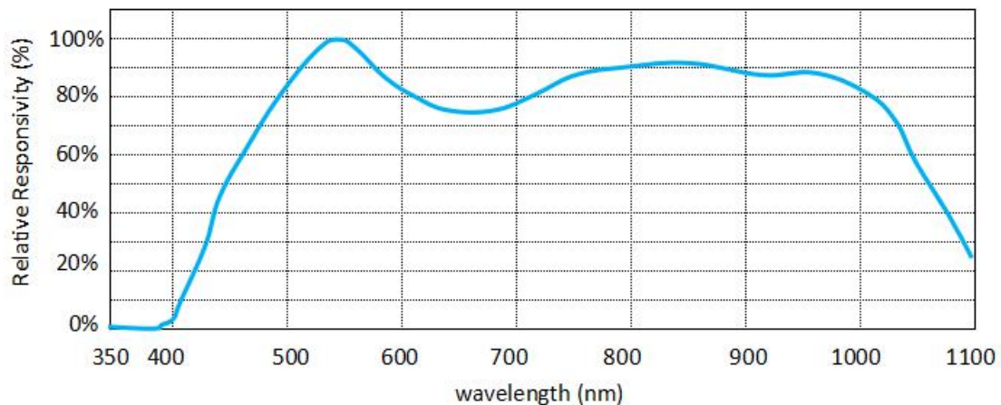
光谱响应度曲线（典型）
