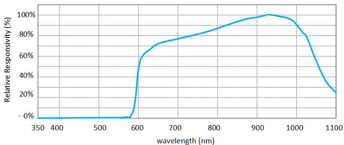
光谱响应度曲线（典型）
